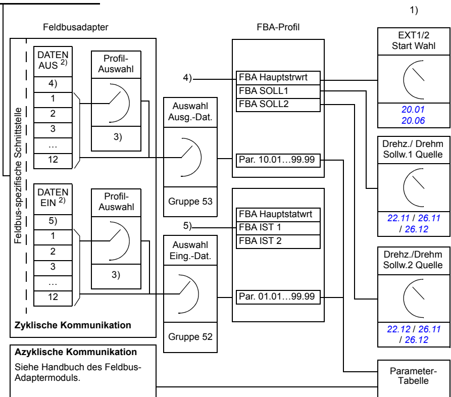
Feldbus-Netzwerk
